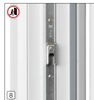
8 incontro antieffrazione presente sulla ferramenta anta secondaria
